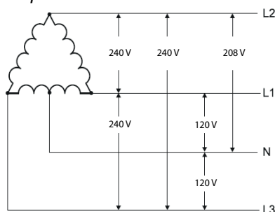
Fig. 4 Système biphasé avec neutre (3 fils)
